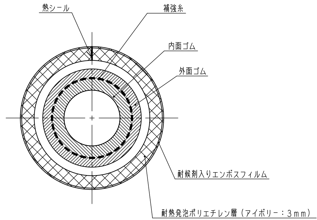
パイプ断面詳細 (S=2:1)
