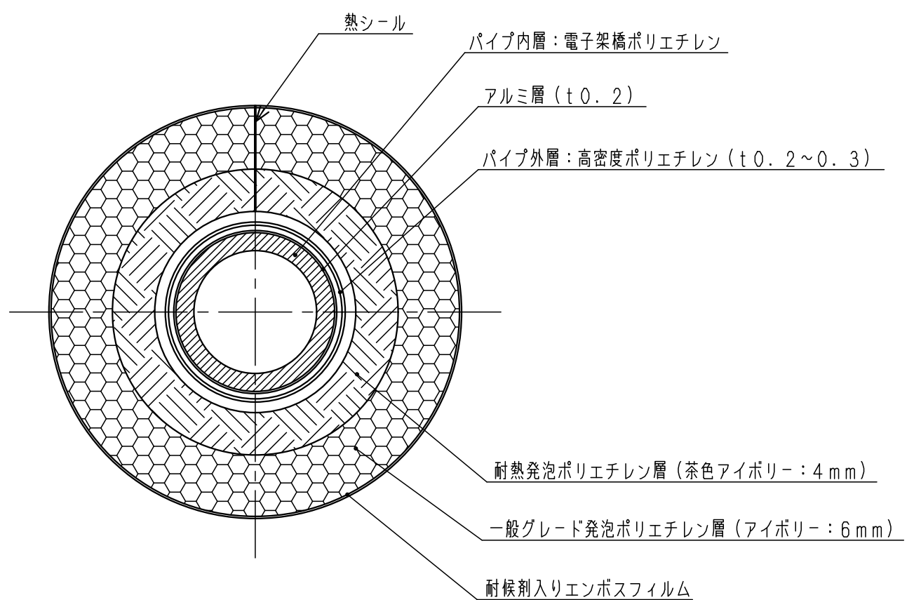
パイプ断面詳細 (S=2:1)
