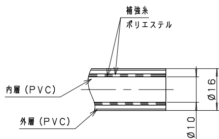
スマートホース \phi 16 断面詳細
