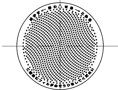
矢視図
